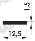
Pr.No: 8592 0,051 kg/m
