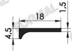
Pr.No.:9809 0,088 kg/m
