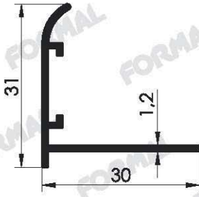
Pr.No:9805 0,223 kg/m
