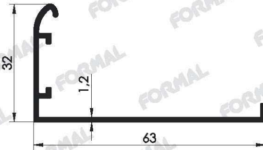
Pr.No: 9112 0,365 kg/m
