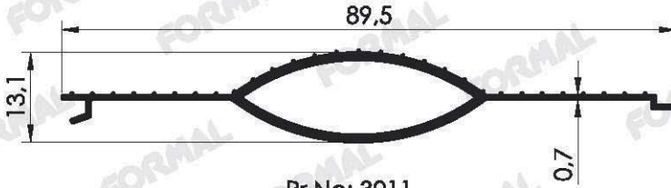
Pr.No: 3011 0,345 kg/m
