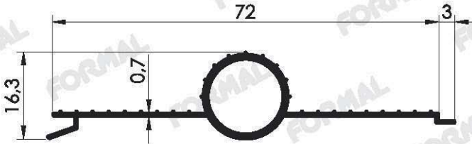
Pr.No: 3009 0,281 kg/m
