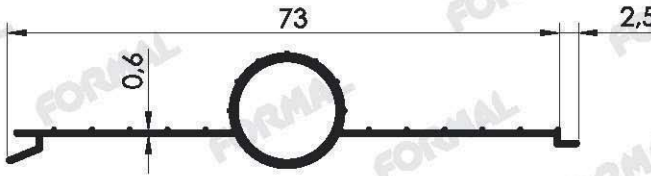
Pr.No : 3042 0,224 kg/m
