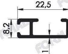
Pr.No: 1289 0,132 kg/m
