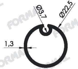
Pr.No: 8856 0,273 kg/m
