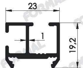
Pr.No: 1331 0,265 kg/m
