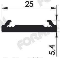
Pr.No: 1334 0,199 kg/m
