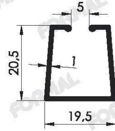
Pr.No: 9130 0,187 kg/m
