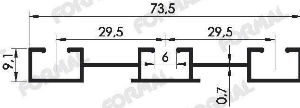
Pr.No: 8054 0,266 kg/m
