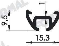
Pr.No: 1288 0,107 kg/m
