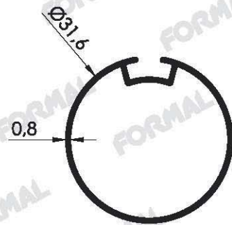
Pr.No: 1676 0,233 kg/m
