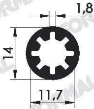
Pr.No: 1678 0,211 kg/m
