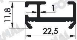
Pr.No: 1333 0,184 kg/m
