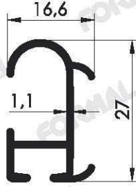
Pr.No: 1086 0,222 kg/m
