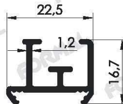
Pr.No: 1332 0,217 kg/m
