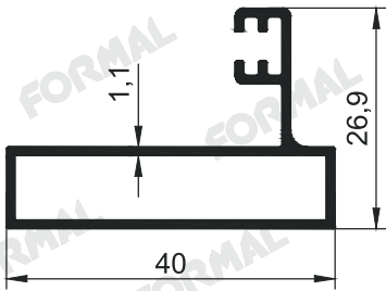
Pr.No: 1816 0,391 kg/m
