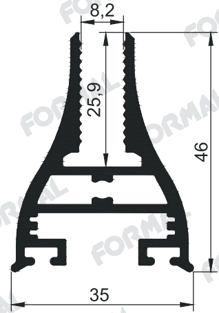
Pr.No: 9620 1,009 kg/m
