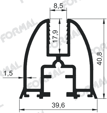
Pr.No: 2219 0,916 kg/m
