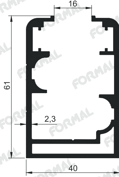
Pr.No: 1814 1,482 kg/m
