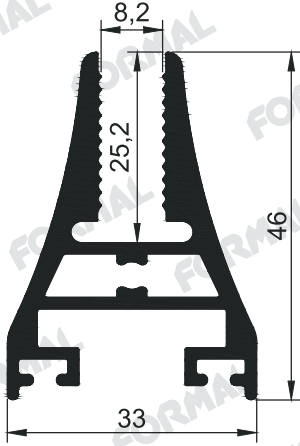
Pr.No: 9308 1,104 kg/m
