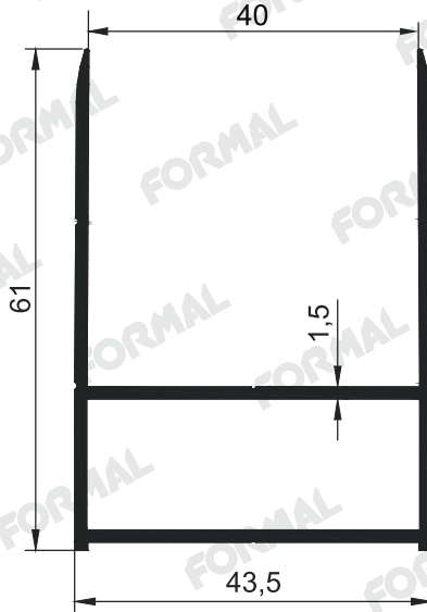
Pr.No: 1817 0,811 kg/m
