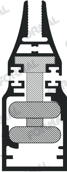
Pr.No: 9308
