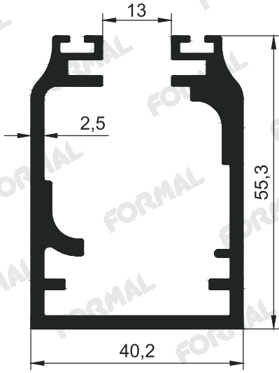
Pr.No: 9307 1,482 kg/m
