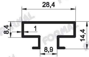
Pr.No: 1036 0,213 kg/m
