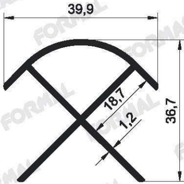
Pr.No: 8149 0,439 kg/m
