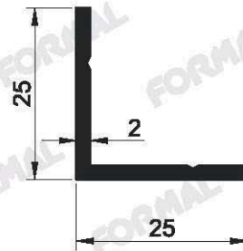
Pr.No: 1224 0,257 kg/m
