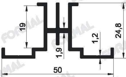
Pr.No: 1621 0,445 kg/m
