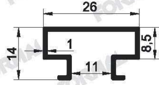
Pr.No: 8791 0,189 kg/m
