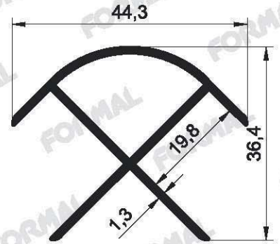
Pr.No: 8596 0,472 kg/m
