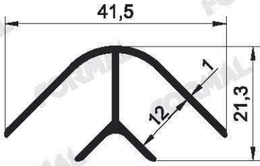
Pr.No: 9744 0,240 kg/m
