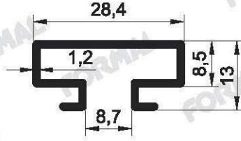
Pr.No: 8148 0,240 kg/m
