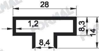
Pr.No: 8151 0,229 kg/m
