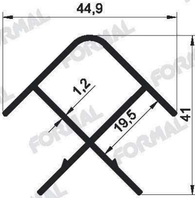
Pr.No: 8801 0,447 kg/m
