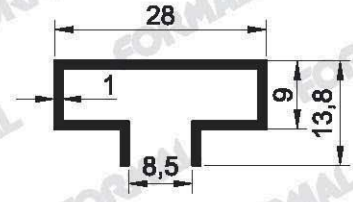
Pr.No: 2158 0,193 kg/m
