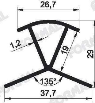
Pr.No: 8933 0,345 kg/m
